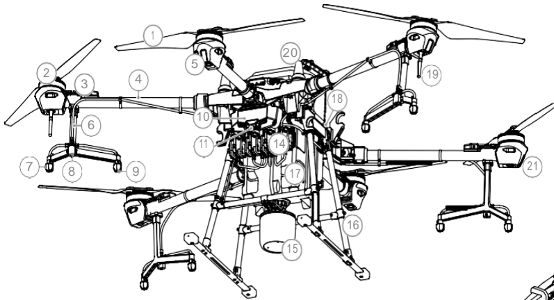
● Вид спереди
